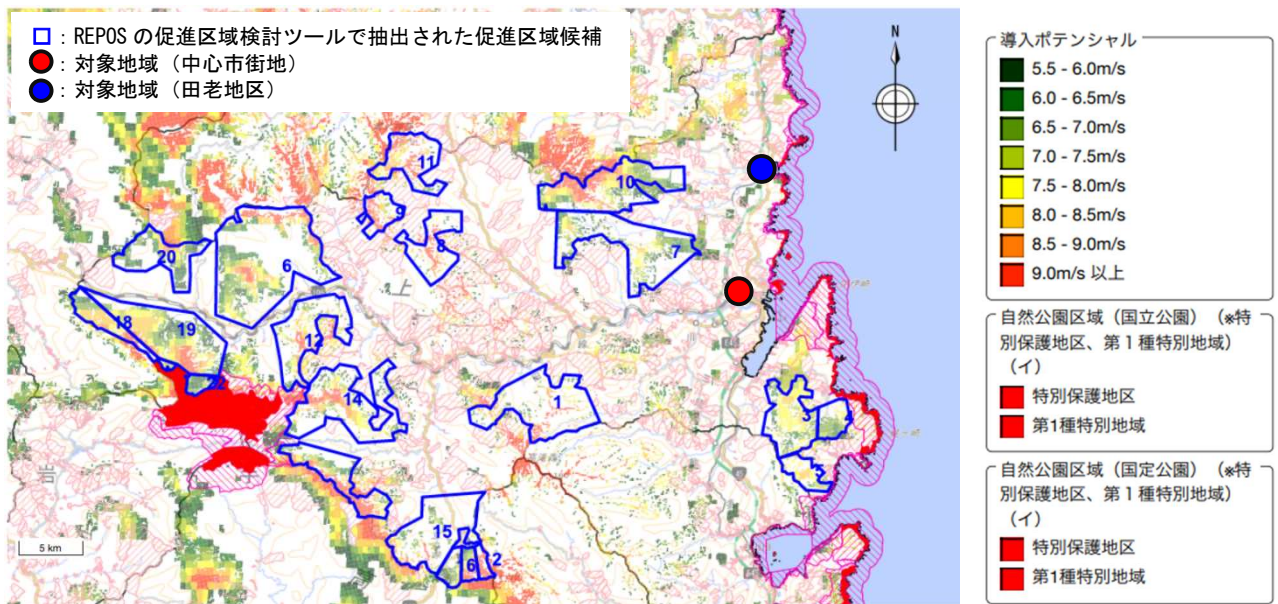
風力発電のポテンシャルマップ（REPOS の促進区域検討支援ツール引用）
