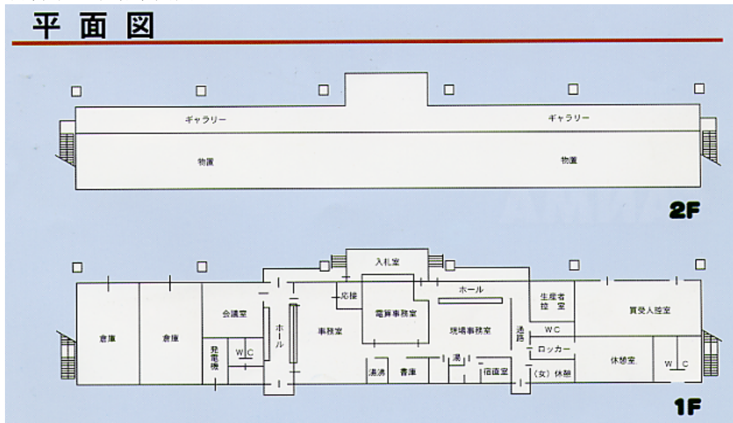
宮古市魚市場平面図
