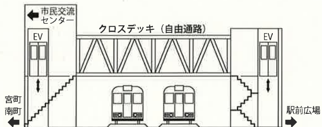
クロスデッキの断面略図。イーストピアみやこに行くためだけでなく、宮町・南町方面と「まちなか」を結ぶ“近道”としても便利です
