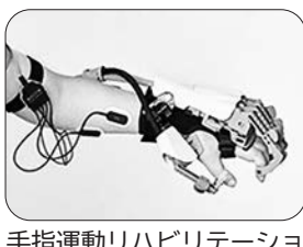
手指運動リハビリテーションシステム
