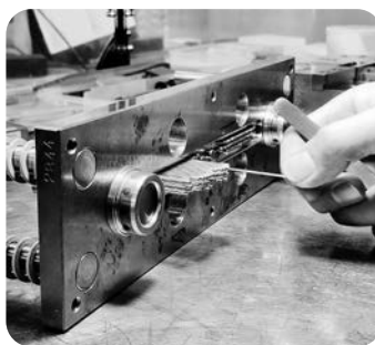
プラスチック成形金型を組み立てる作業
