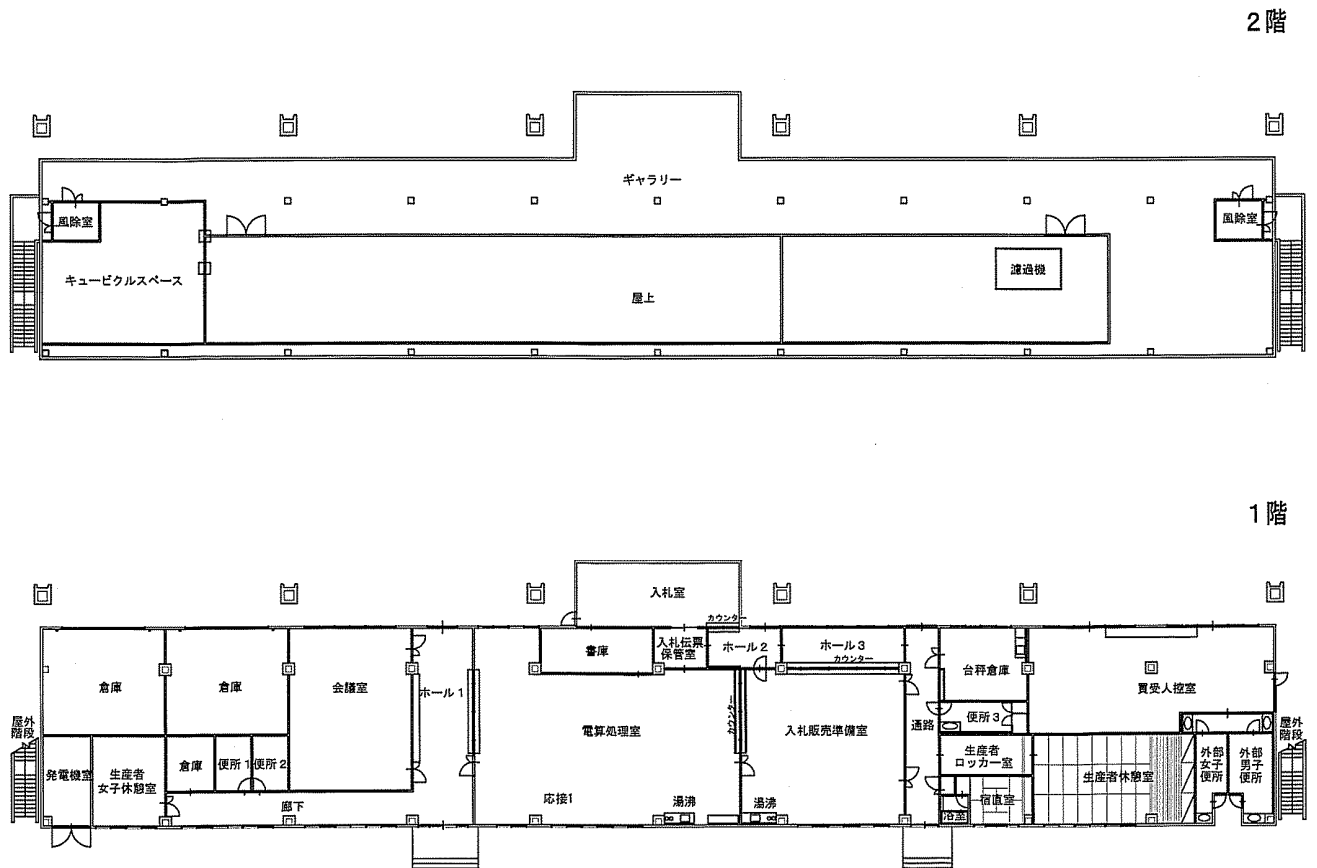
宮古市魚市場平面図
