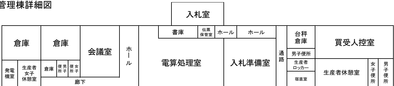
管理棟詳細図
