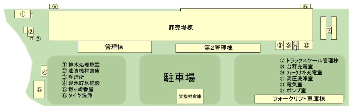
宮古市魚市場全体図
