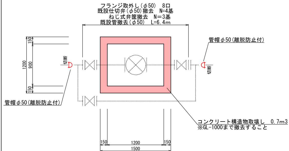
減圧弁取壊し詳細図
