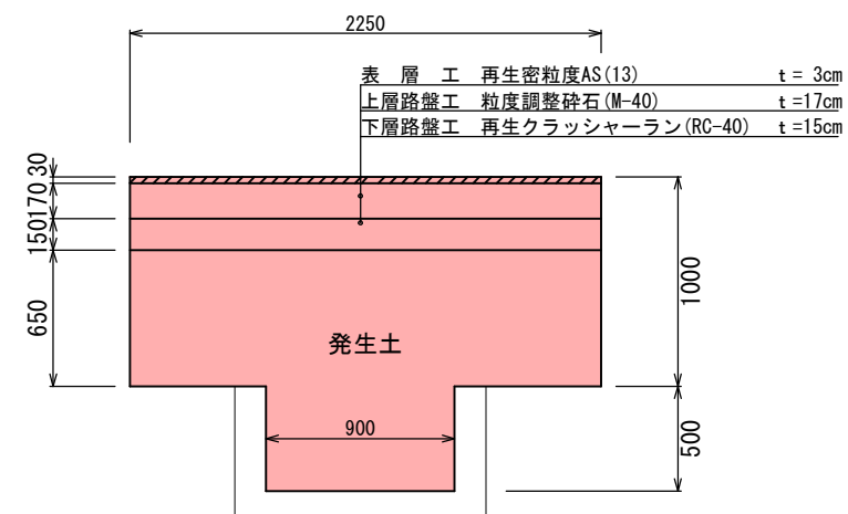
減圧弁撤去土工断面図 (仮復旧)
