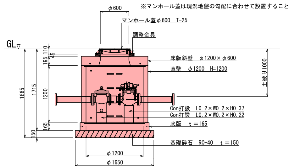
2号マンホール詳細図
