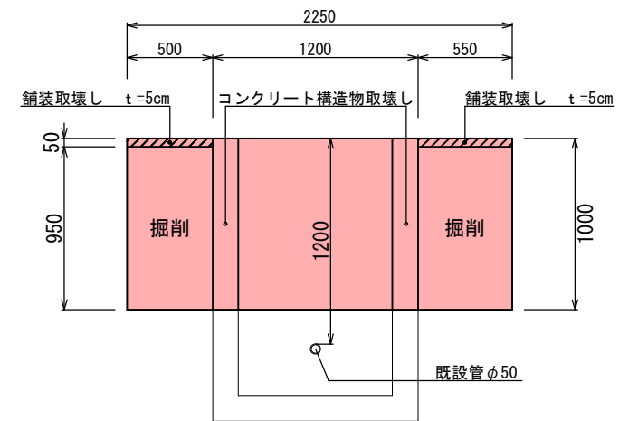
減圧弁撤去土工断面図 (仮復旧)
