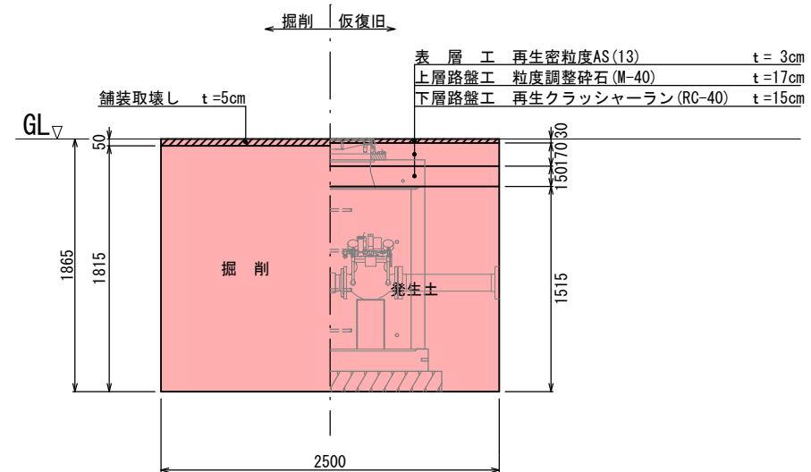
減圧弁撤去詳細図
