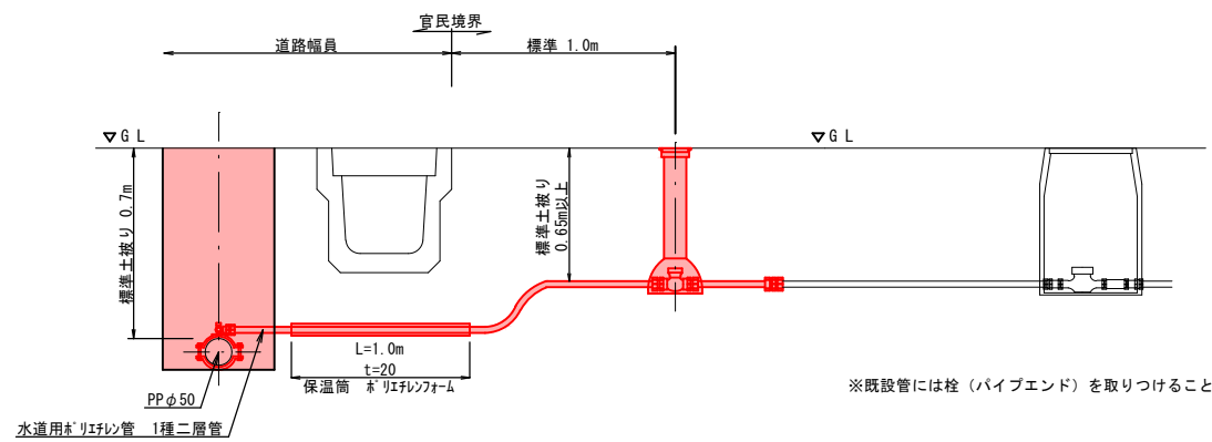
給水切替工標準図 S=FREE
