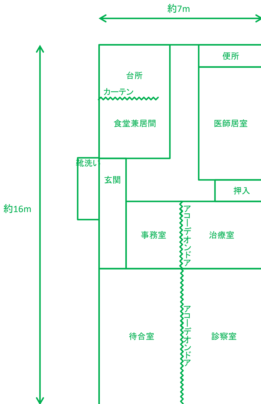
(4) 避難所 レイアウト図 (2/2)
