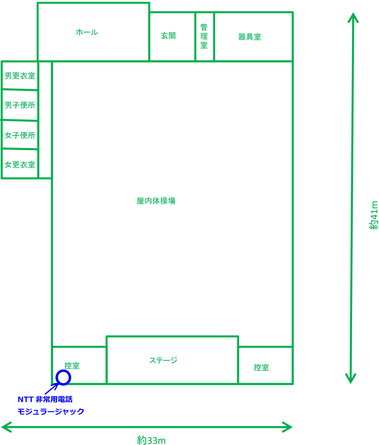
1 階 平 面 図
