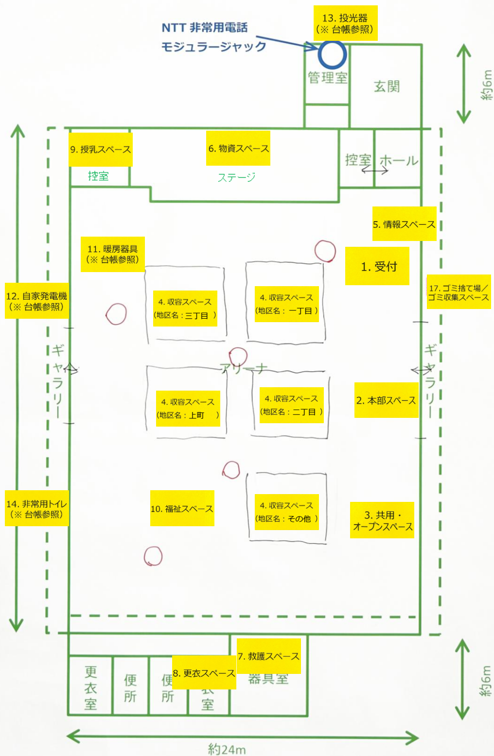
1 階 平 面 図
