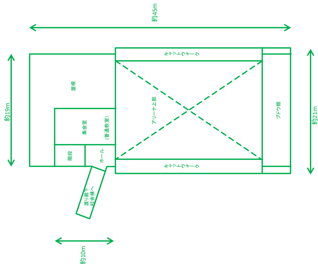
管理教室棟・屋内運動場 2 階 平面図
