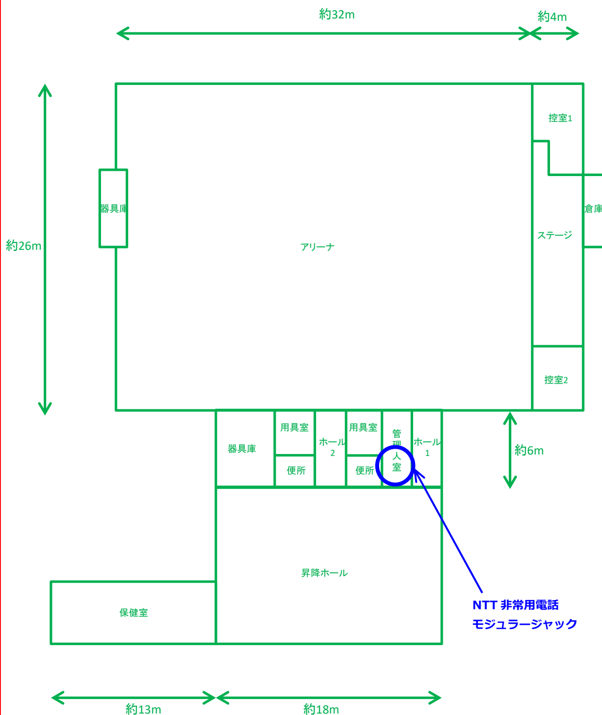
屋内運動場 1 階 平面図
