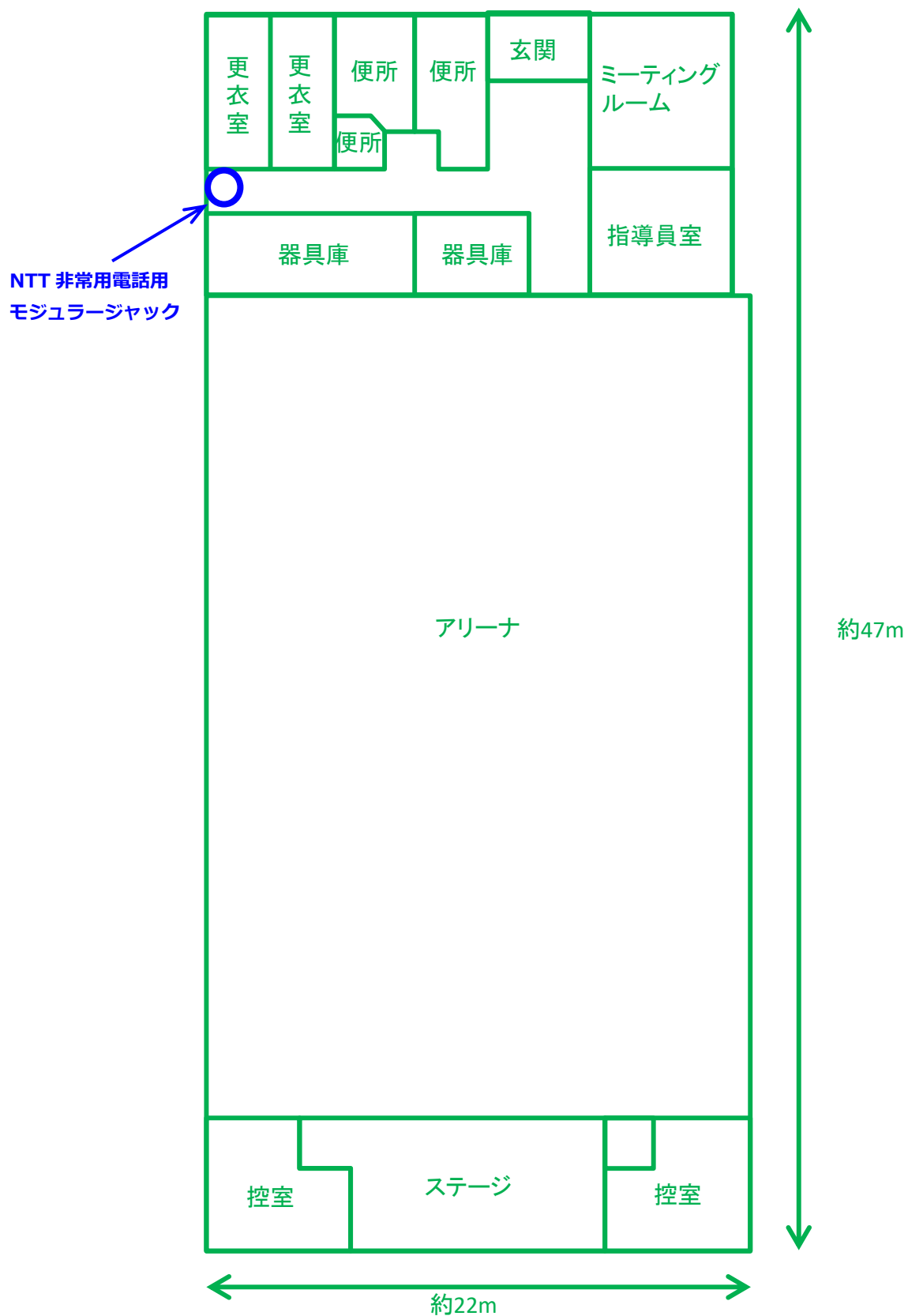
1 階 平 面 図
