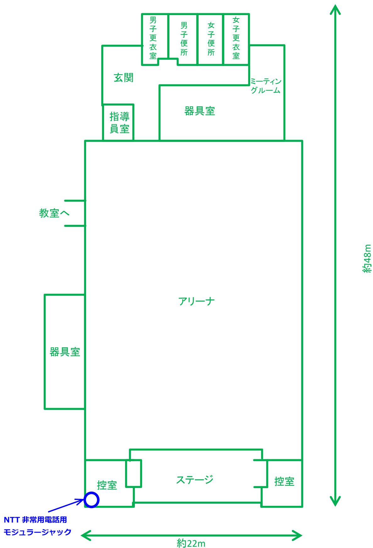
1 階 平 面 図
