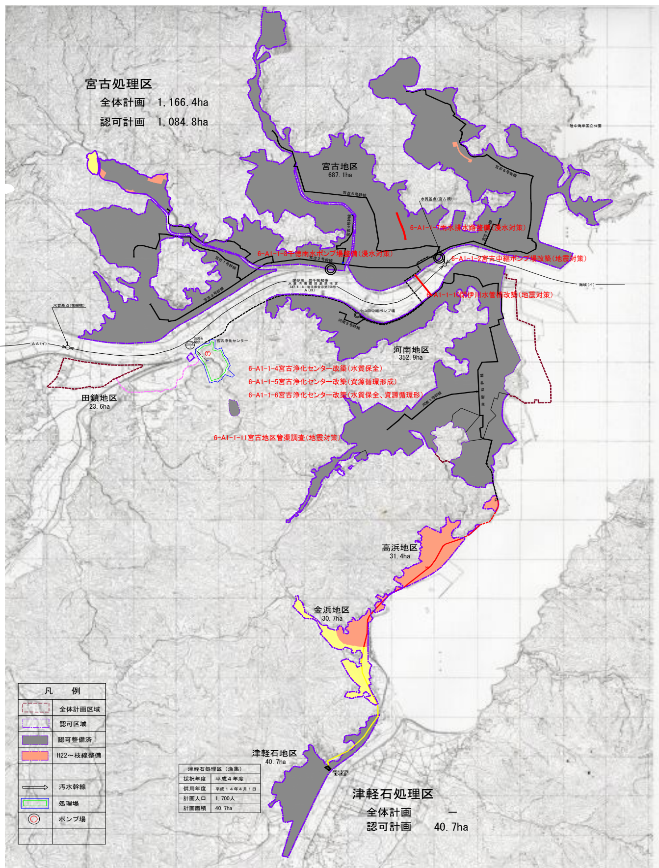
宮古処理区計画図
