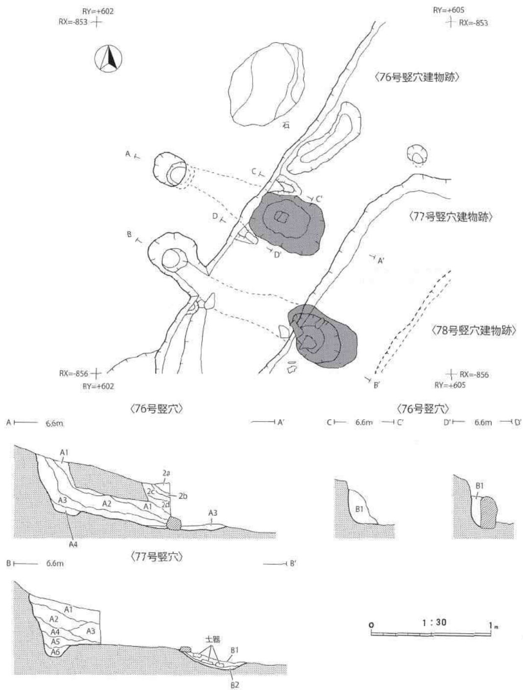
第 188 図 76 号・77 号竖穴建物跡 カマド 平面図・断面図
