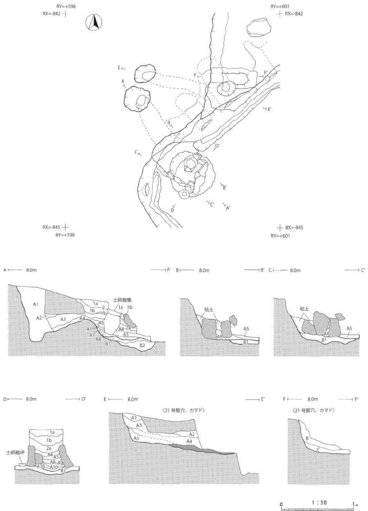
第 133 図 4 号・21 号竪穴建物跡 カマド 平面図・断面図
