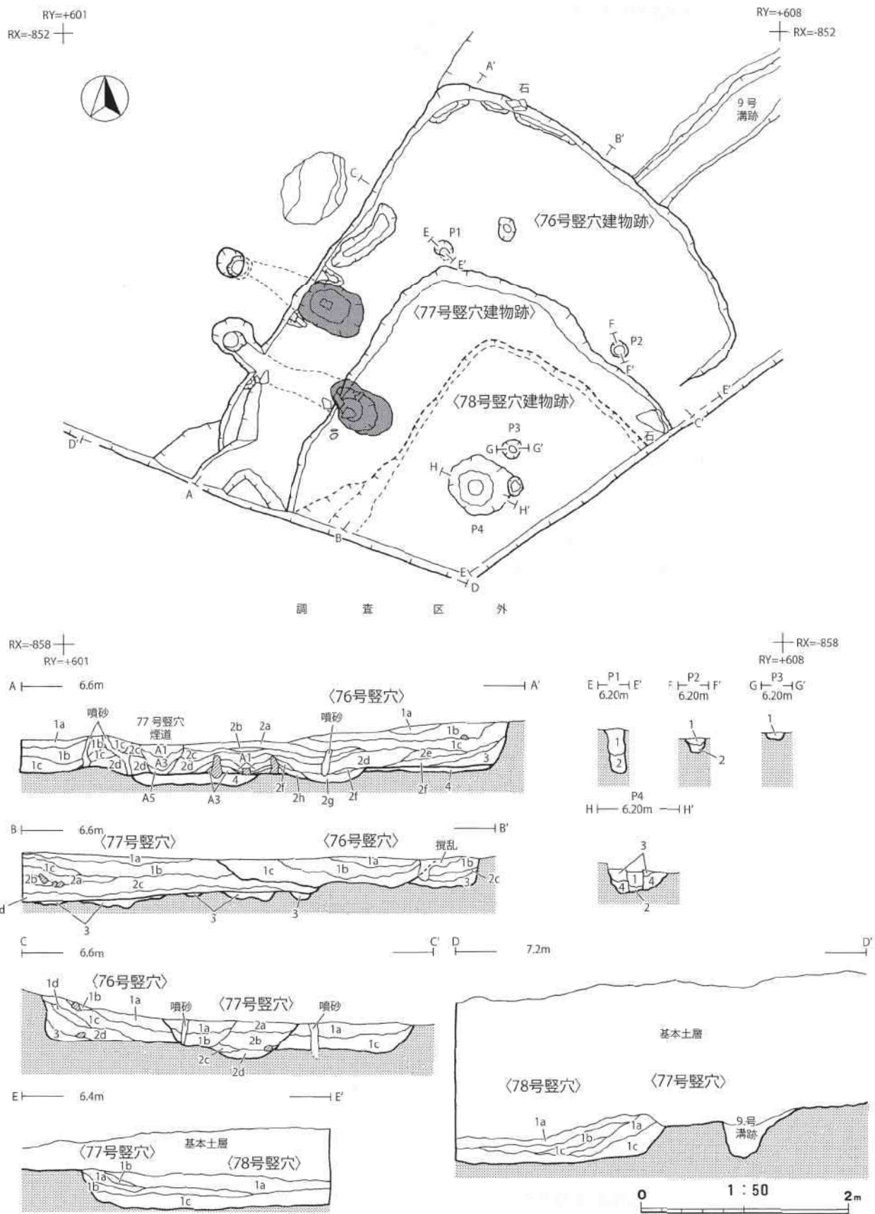
第187図 76号竖穴建物跡 平面図・断面図
