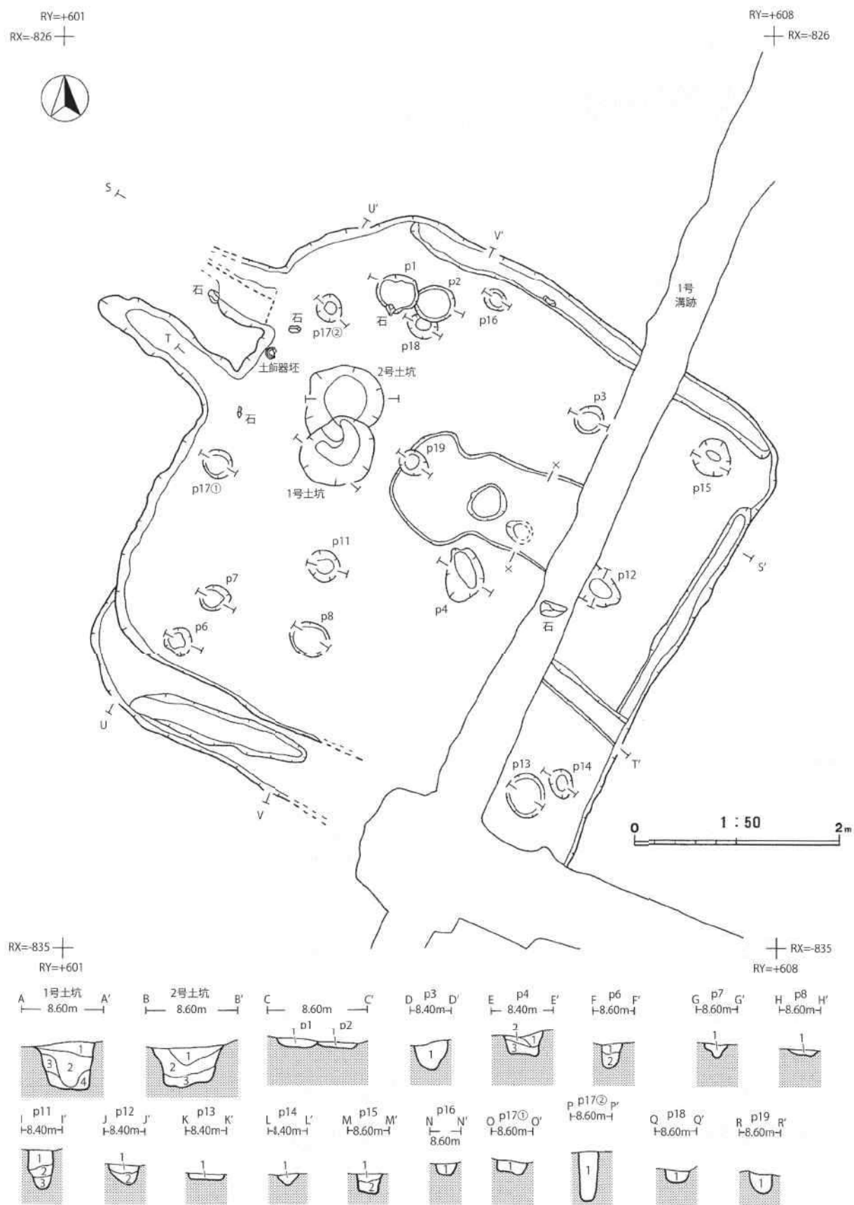
第 170 图 31 号竖穴建物跡 平面図・断面図
