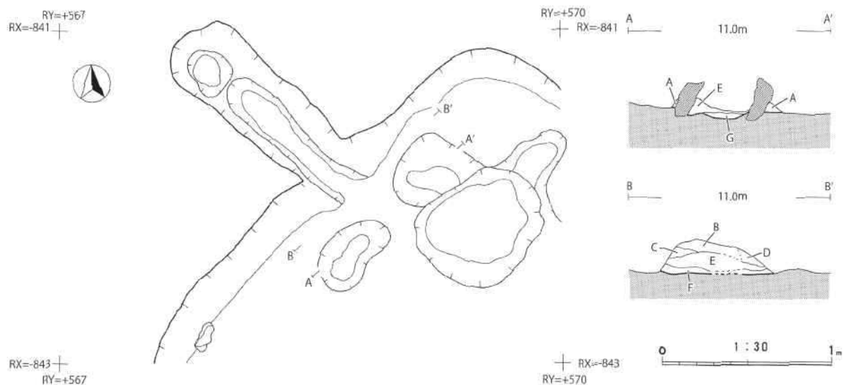
第 140 図 30 号竪穴建物跡 カマド② 平面図・断面図 (2)
