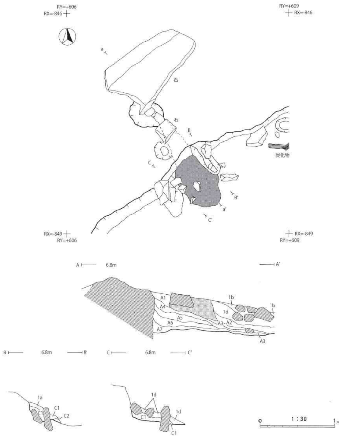
第 186 図 63 号竪穴建物跡 カマド 平面図・断面図
